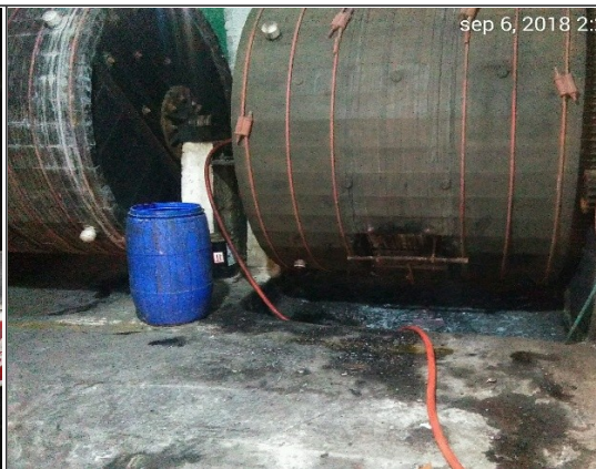
Foto No. 4 Bombo cargado, proceso de curtido vegetal
